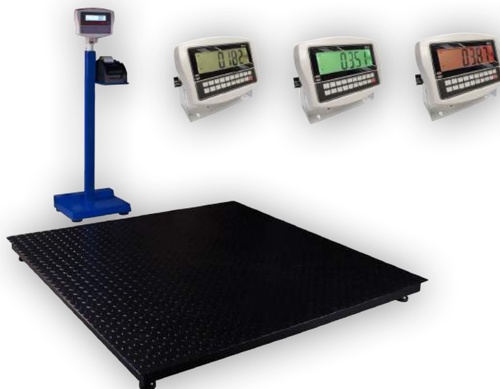
Riba plateauweger met indicator
