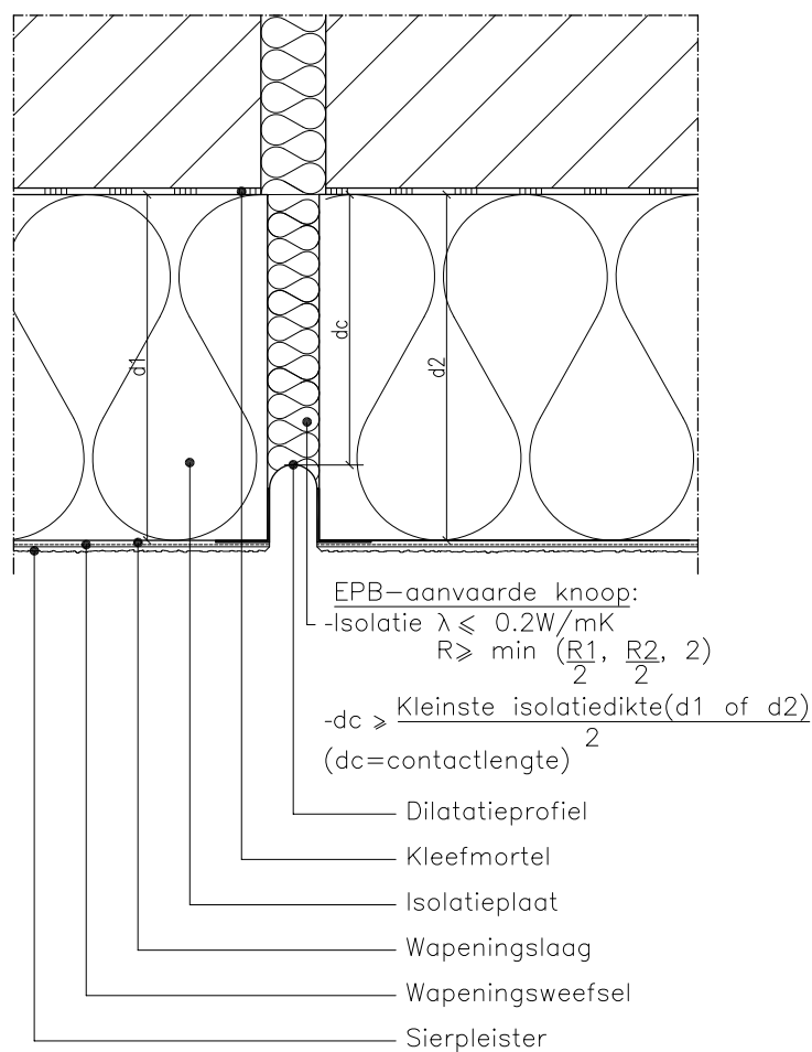
Afb. 17: Uitzettingsvoeg in een hoek
