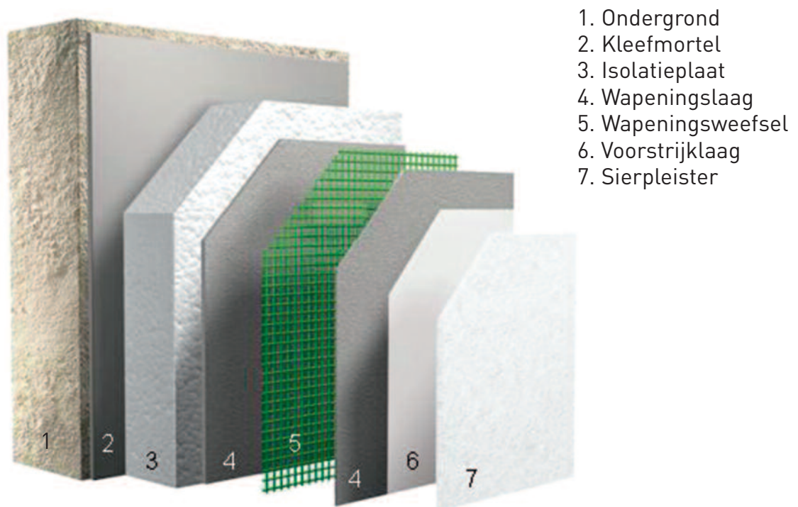
Afb. 10: Systeemopbouw
