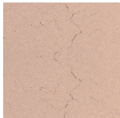
Afb. 25: Krimpscheuren
