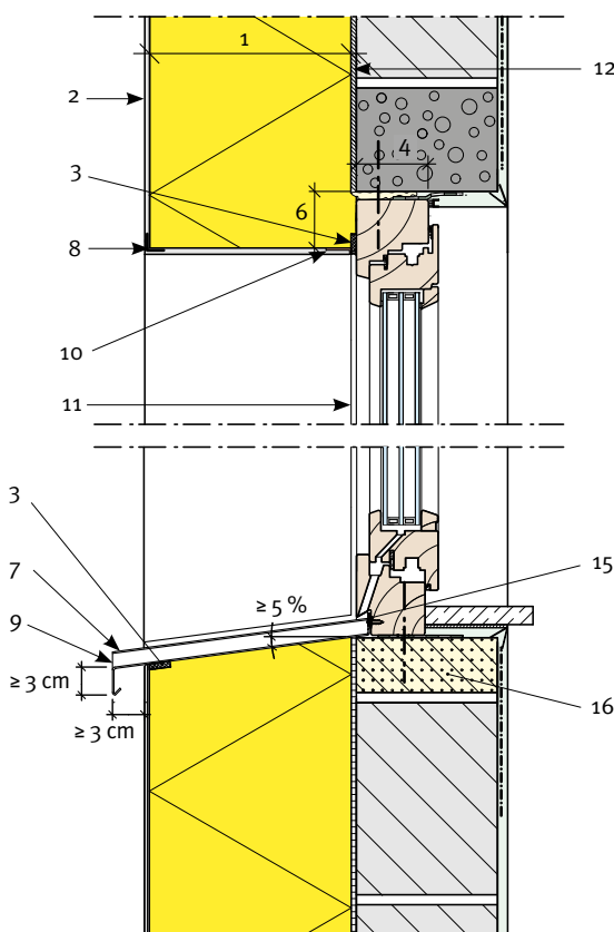
Afb. 60 Aansluiting tussen ETICS en een kader geplaatst op een thermisch isolerend bouwblok (weinig lawaaijerige omgeving).
