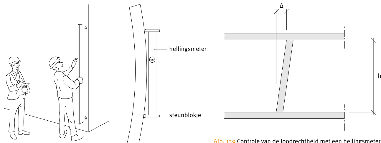
Afb. 139 Controle van de loodrechtheid met een hellingsmeter.
