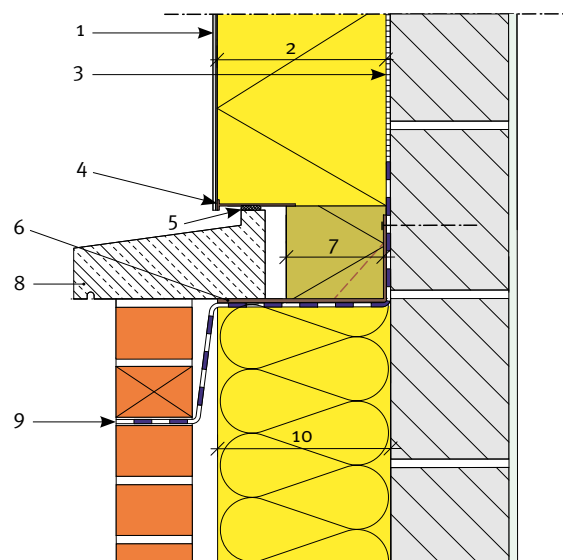
B. Ondersteuning van de muurkap door middel van punctuele versterkingshaken
