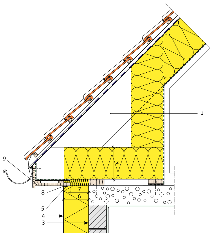
Afb. 75 Aansluiting van een ETICS aan de onderrand van het dakvlak van een hellend dak (geval waarbij het ETICS doorloopt tot tegen bekleding van de dakoversteek).
