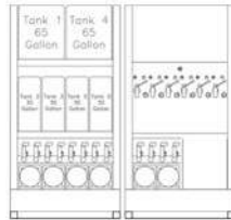
SIZE: 2 x 65 Gallon x 4 x 30 Gallon 92"(w) x 46"(d) x 88"(h)
