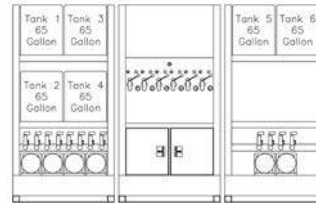
SIZE: 6 x 65 Gallon 138"(w) x 46"(d) x 88"(h)
