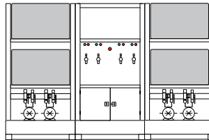
SIZE: 4 x 120 Gallon 138"(w) x 46"(d) x 88"(h)
