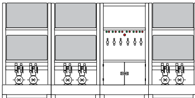
SIZE: 6 x 120 Gallon 184"(w) x 46"(d) x 88"(h)
