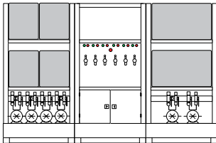
SIZE: 4 x 65 Gallon x 2 x 120 Gallon 138"(w) x 46"(d) x 88"(h)
