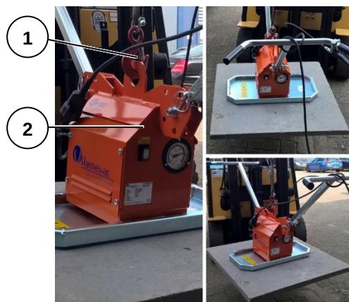
Abbildung 10: Befestigung an der Maschine (Beispiel)
