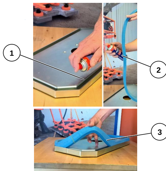
Abbildung 16: Einsetzen des Saugnapfgummis
