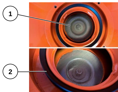
Abbildung 14: Reinigen des Filters
