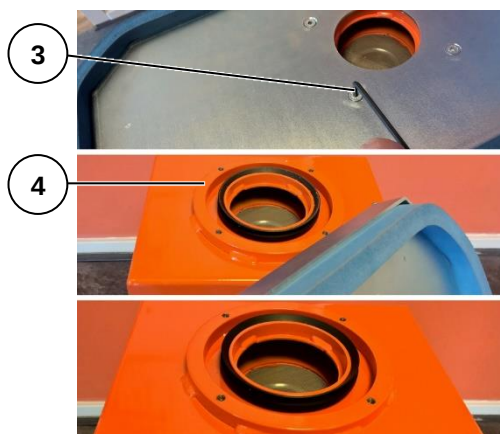
Abbildung 12: Saugnapf wechseln
