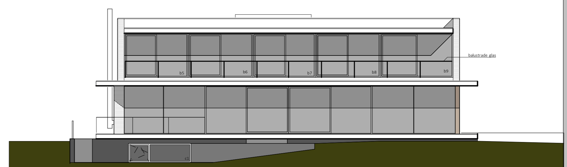
ACHTERGEVEL
