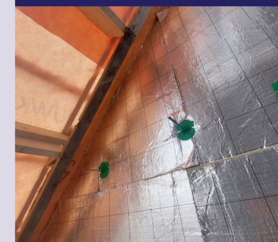
Foto aansluiting isolatie op dak.
