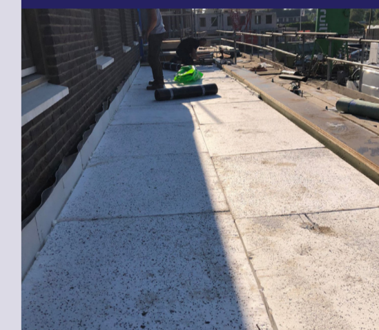
Overzichtsfoto waarop gehele dak te zien is.
