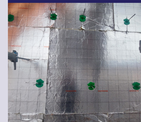
Foto's waarop aansluiting isolatiemateriaal op elkaar.
